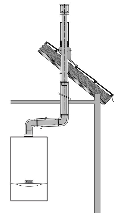
Пример комплекта дымоходов для turboTEC
