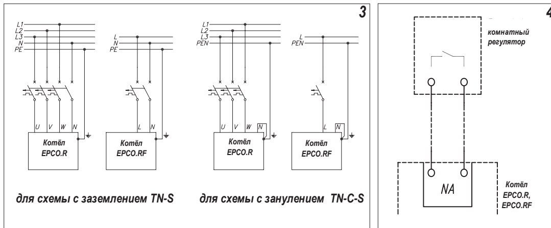
Рис.3 Подключение к электрической проводке F - сетевой выключатель
