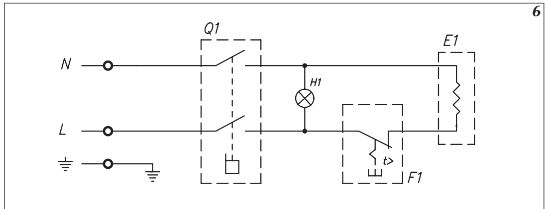
Рис.6 Принципиальная схема
